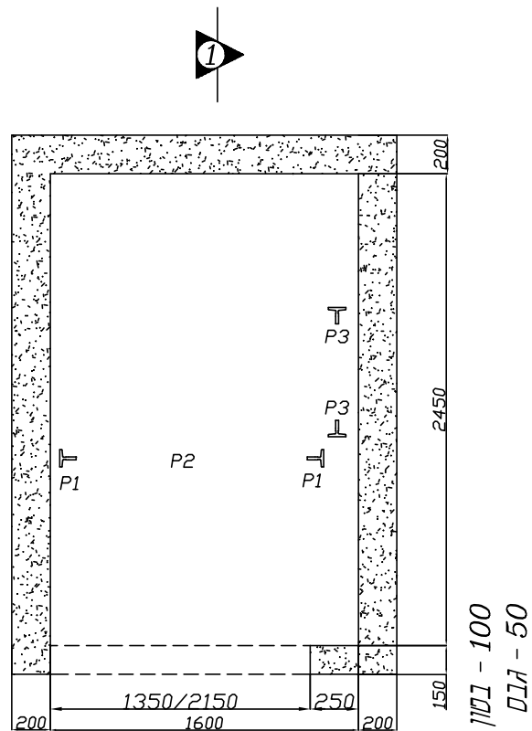
תחנה תחתונה
