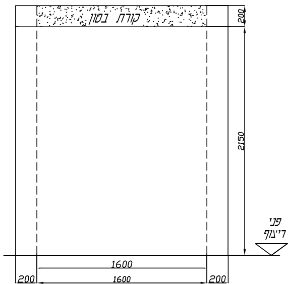
מבט חזית - תחנה עליונה
