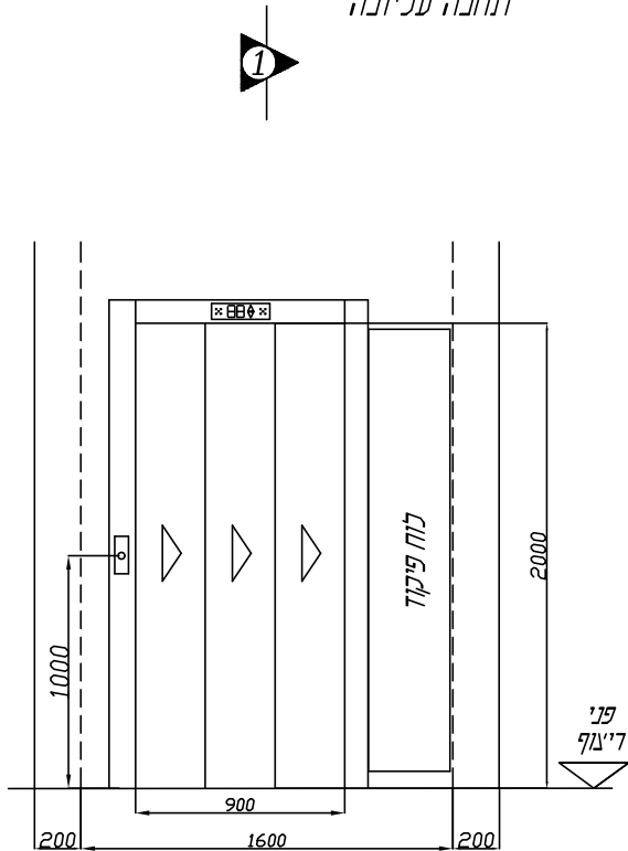
מבט חזית - תחנה עליונה
