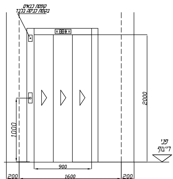
מבט חזית - תחנה תחתונה
