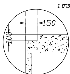
פרט רצפה ללא ריצוף
