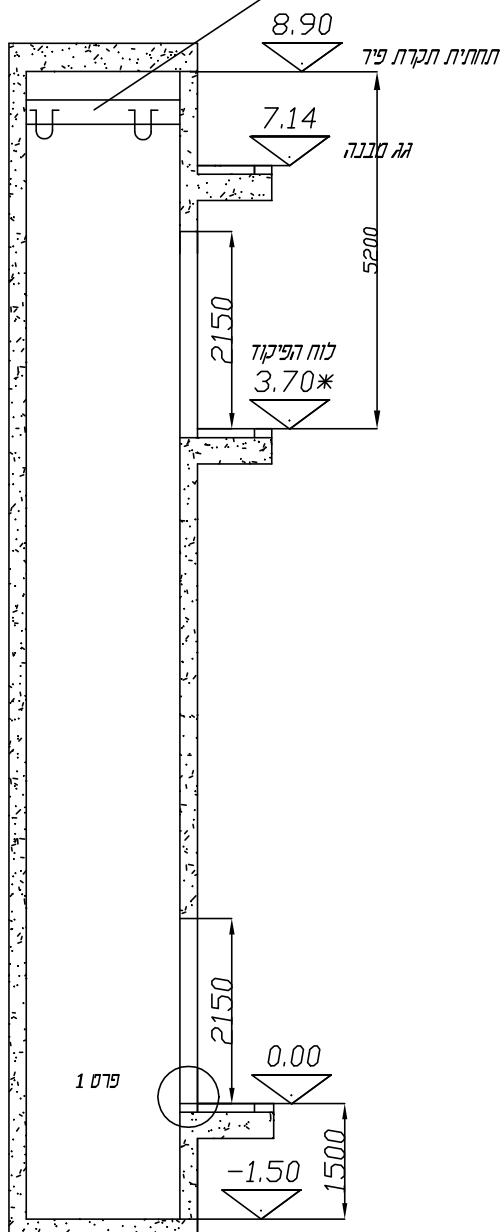
חתך 1-1 תכנית בניה
