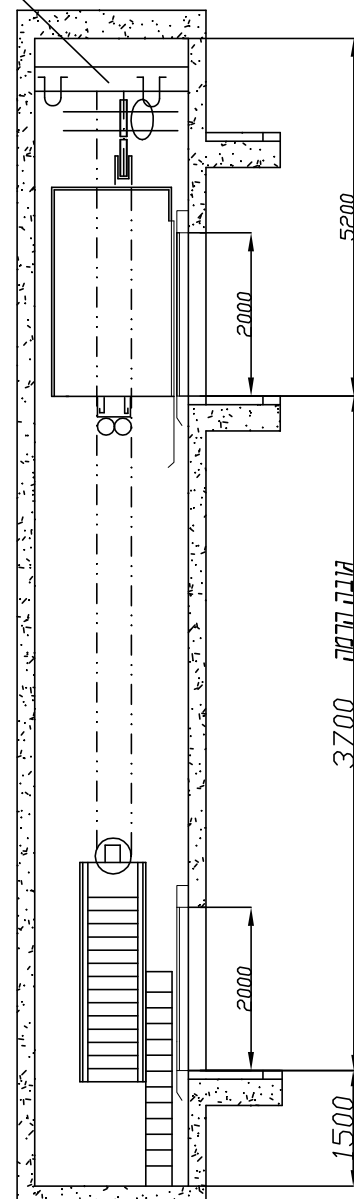
חתך 1-1 תכנית הרכבה
