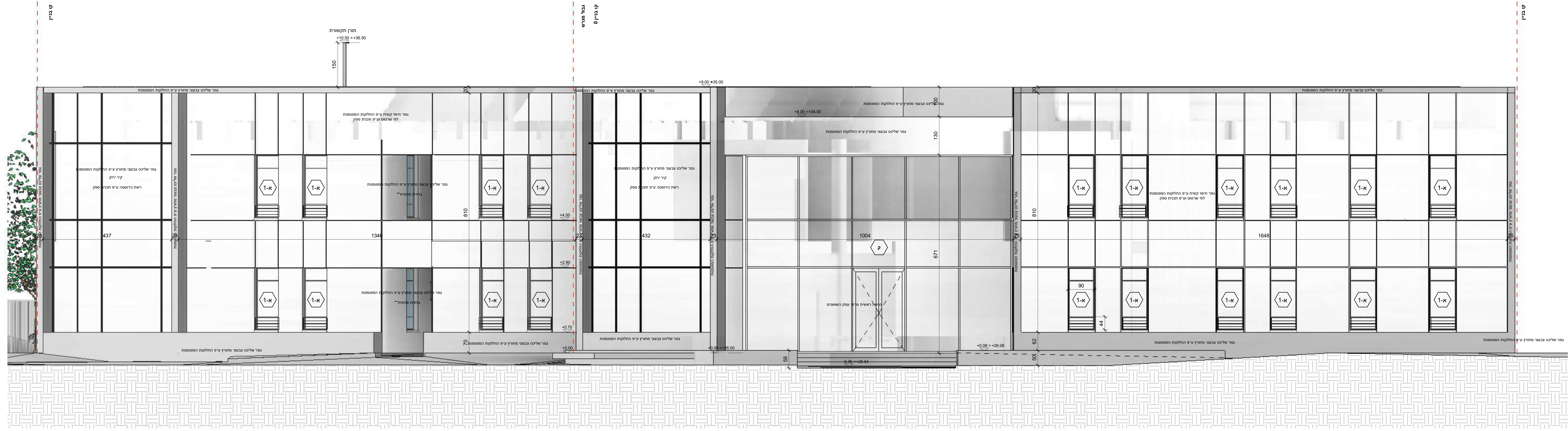
חזית דרומית W 1 : 50 ①
