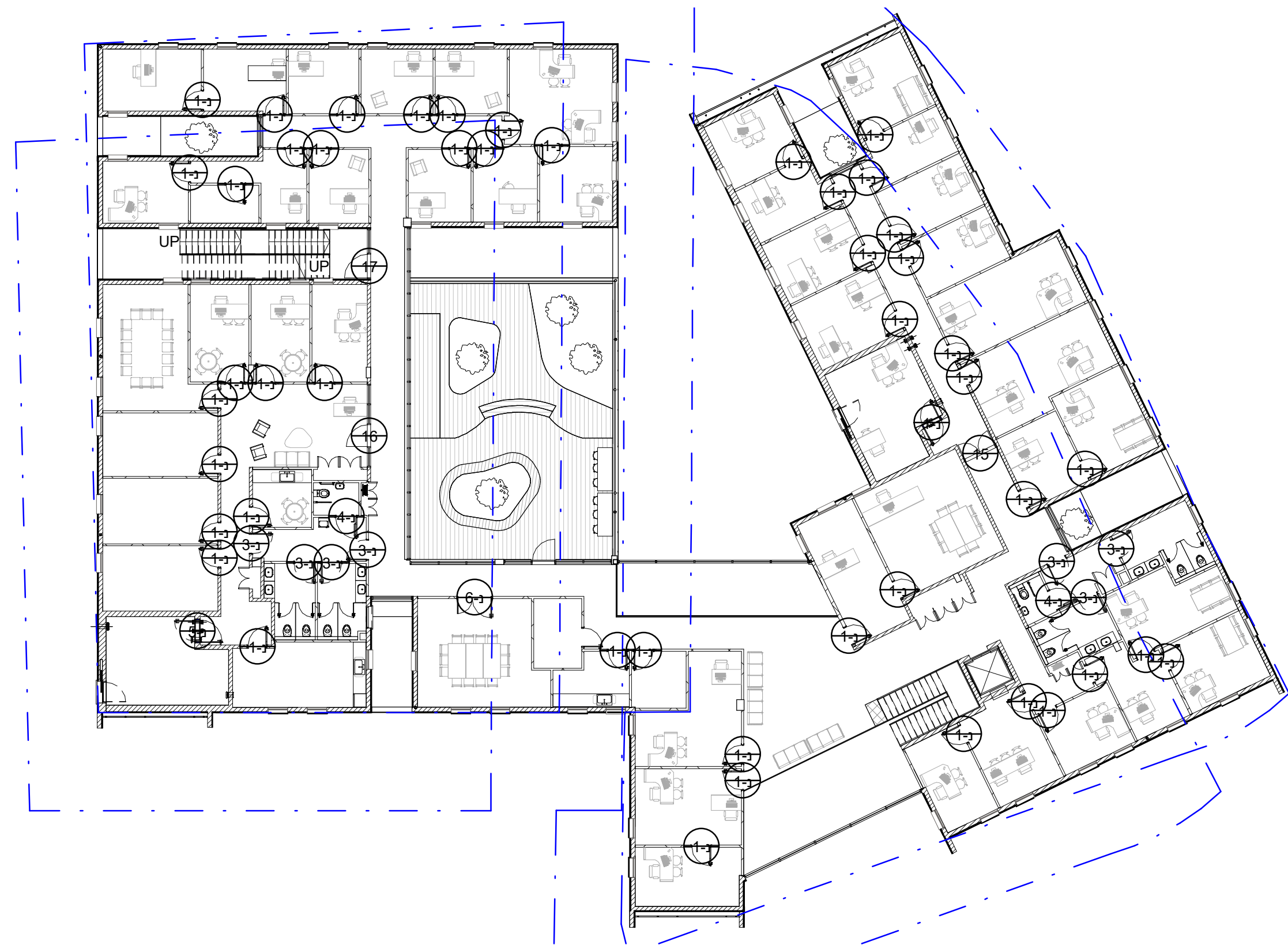
קומה ראשונה לרשימת נגרות 1 : 200
