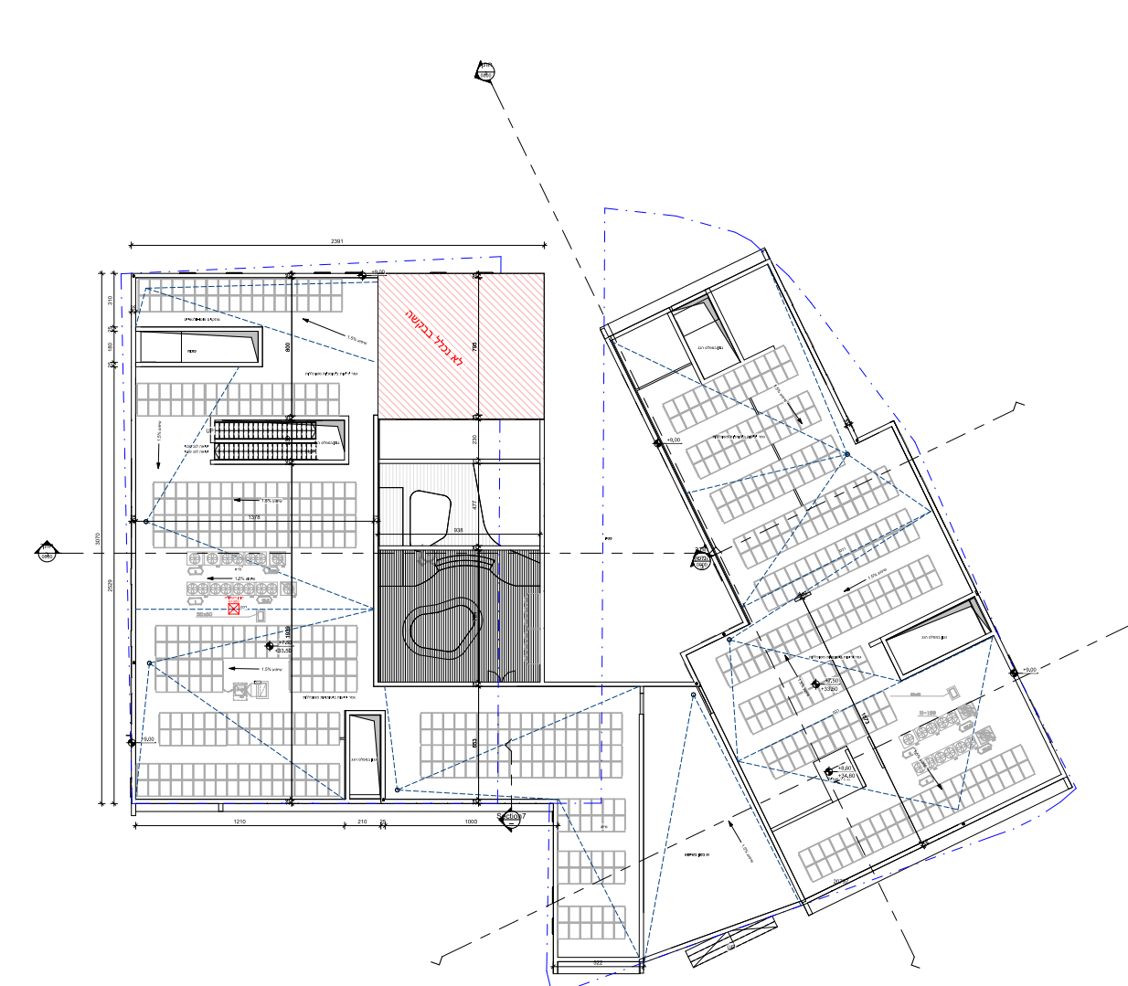
3 תכנית בגוף 1:100
