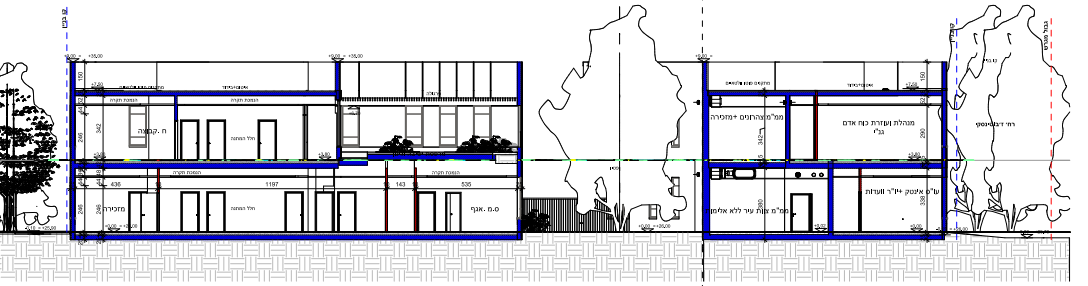
6 חתך ב' 1:100
