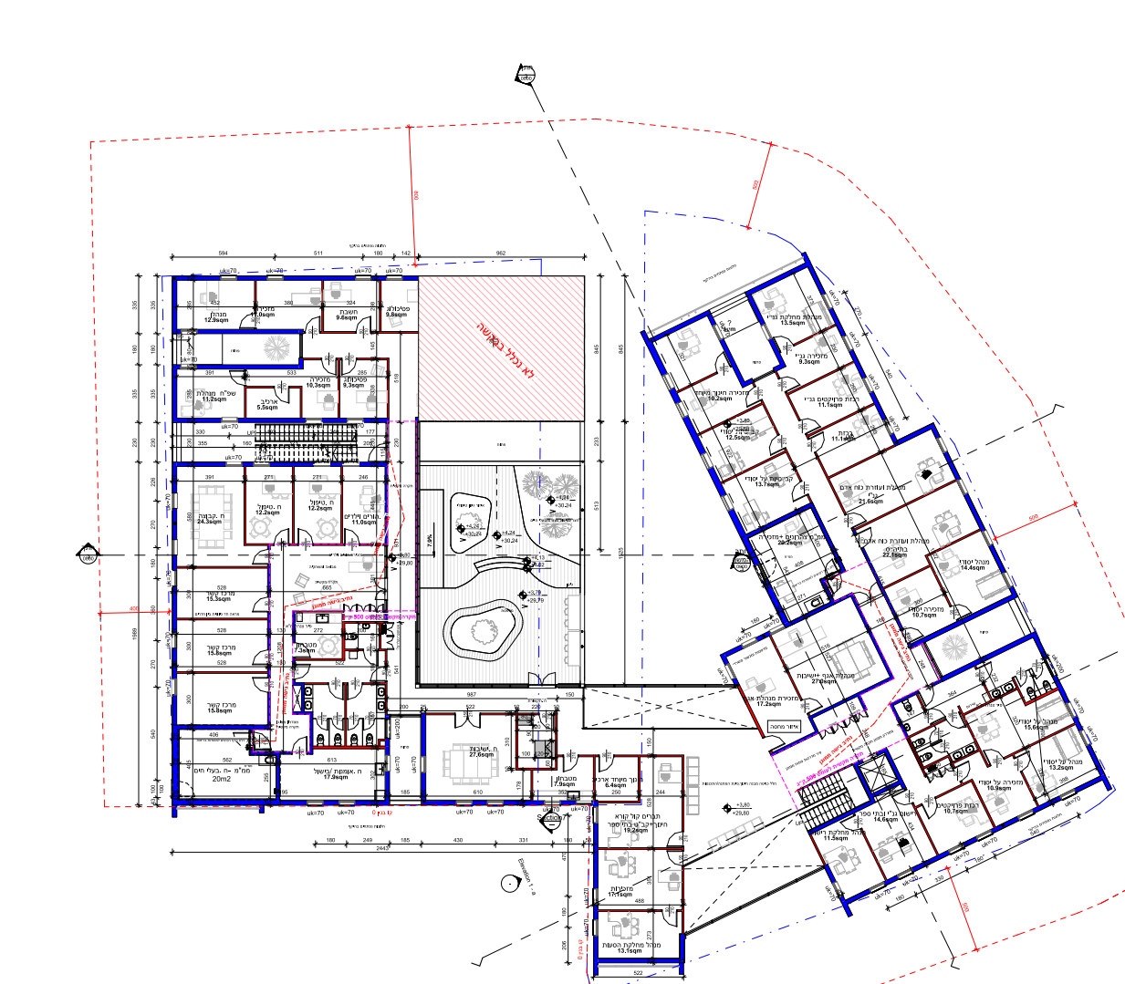
2 קומה ראשונה 1:100
