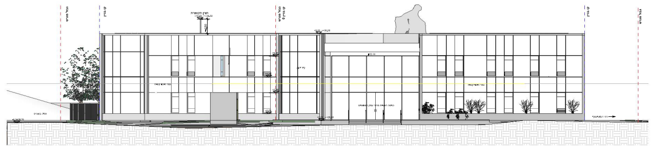
8 חזית דרומית 1:100
