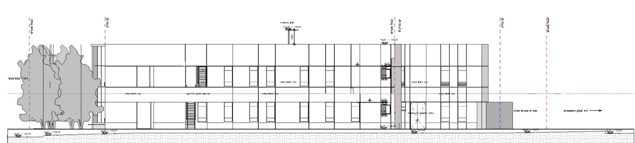
10 חזית מערבית 1:100
