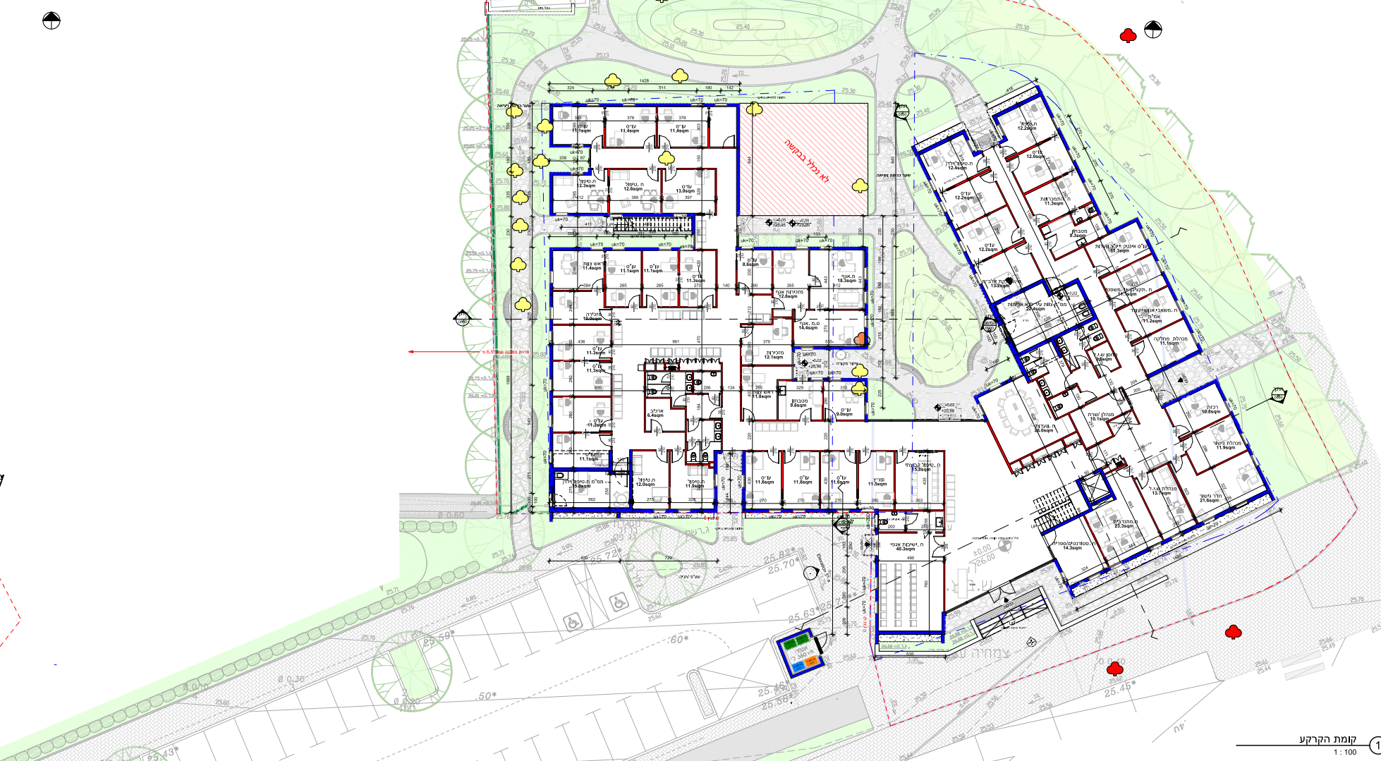
1 קומת הקרקע 1:100
