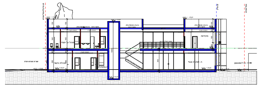
4 חתך א' 1:100
