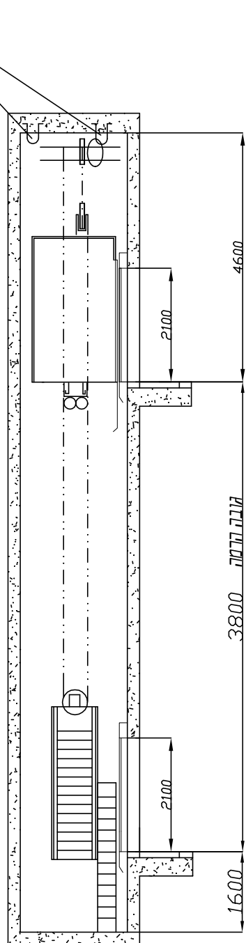
1-1 חתך תכנית הרכבה
