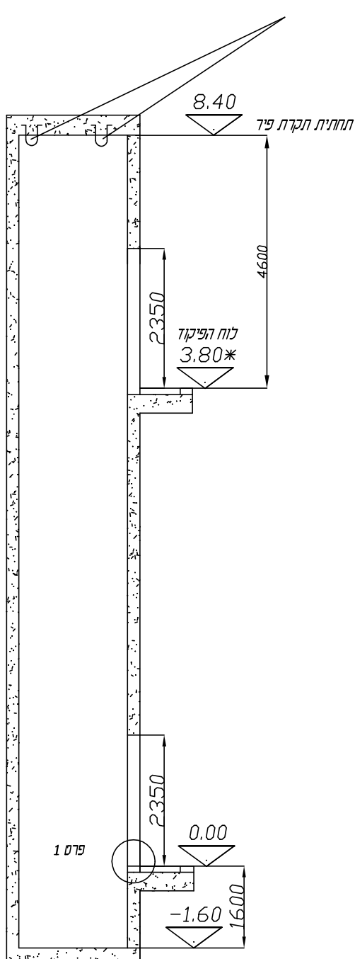
1-1 חתך תכנית בניה
