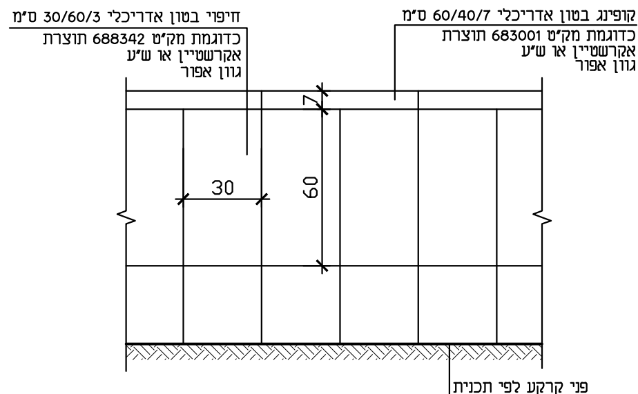
חזית טיפוסית קנ"מ 1:20
