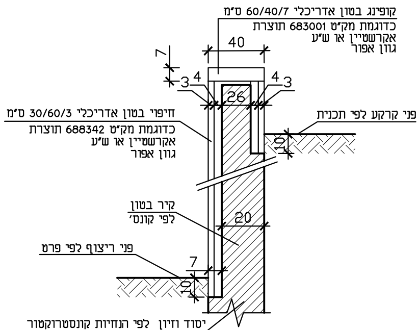
חזת טיפוסית קנ"מ 1:20
