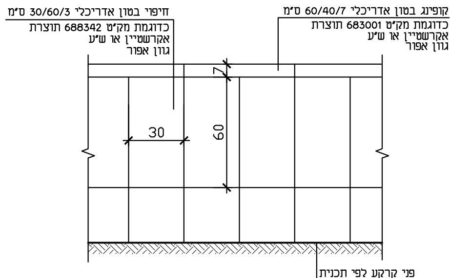
חזית טיפוסי קנ"מ 1:20
