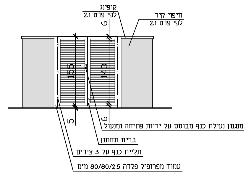
חזית קנ"מ 1:50
