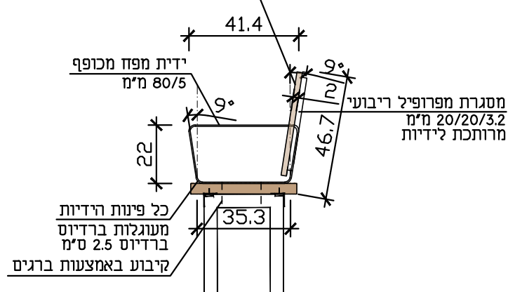
חיתך טיפוסי
