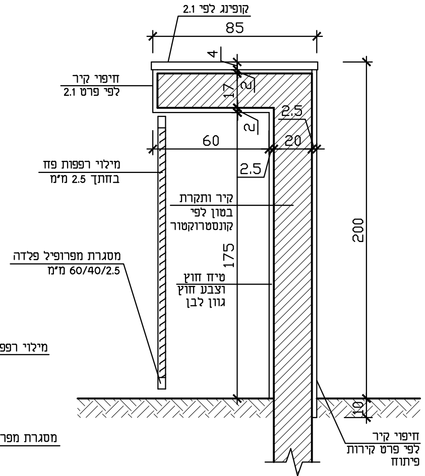
חתך קנ״מ 1:20
