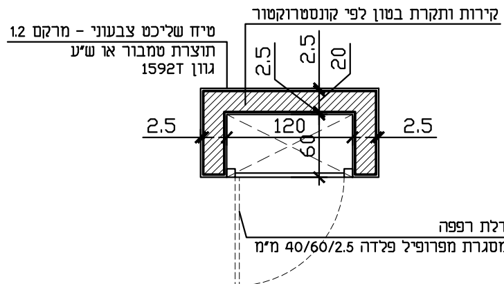
תכנית קנ"מ 1:50
