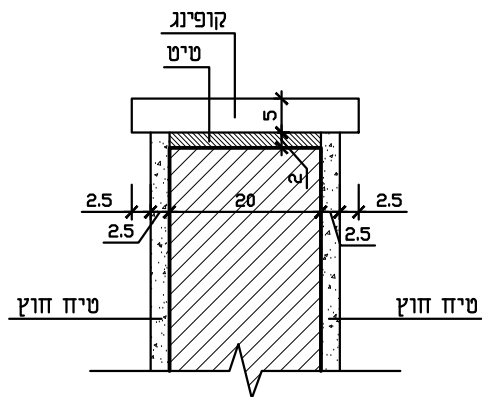
הגדלה ראש קיר קנ"מ 1:10
