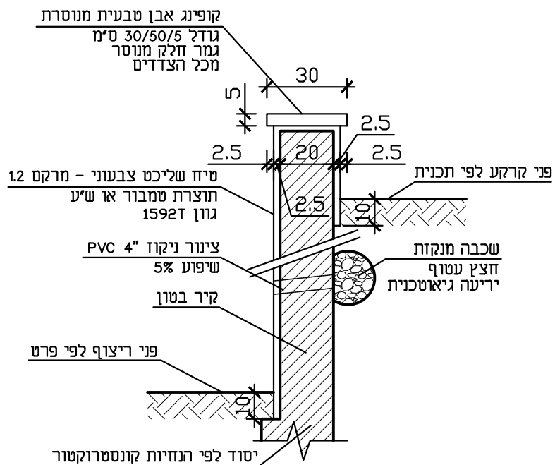
חתך טיפוסי קנ"מ 1:20
