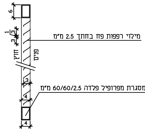
פרט רפפה קנ״מ 1:10
