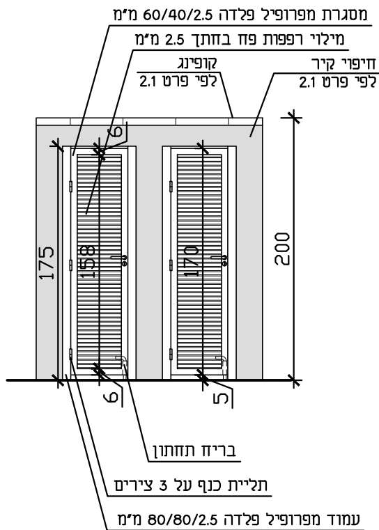
חזית קנ״מ 1:50
