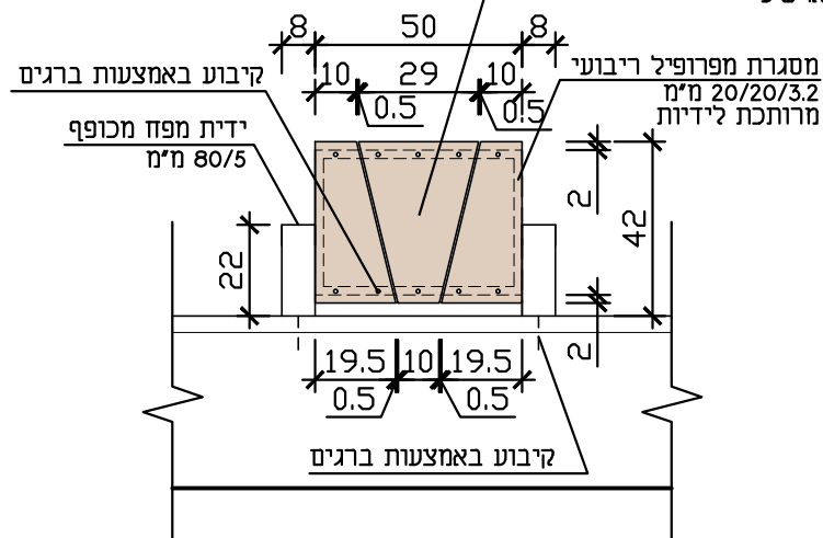
חזית טיפוסית
