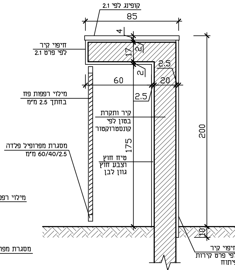
חתך קנ"מ 1:20
