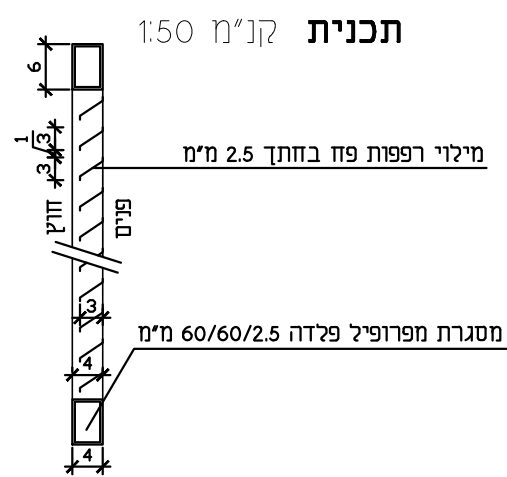
פרט רפפה קנ"מ 1:10
