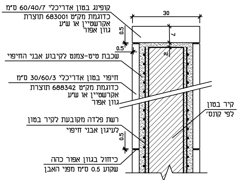
הגדלה ראש קיר קנ"מ 1:10
