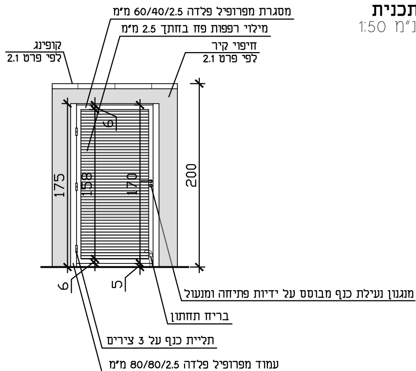
חזית קנ"מ 1:50
