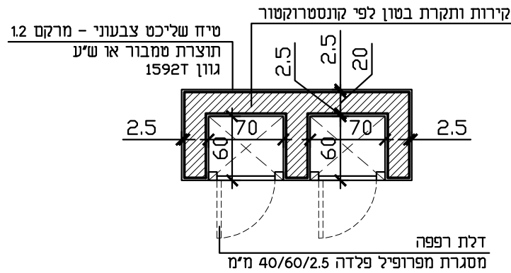
תכנית קנ״מ 1:50
